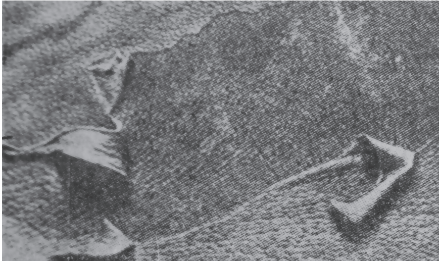
Il. 3. Oddzielanie się lica skóry spowodowane zbyt intensywnym procesem wytrawiania skóry, za: Z. Kowalski, Uszkodzenia i wady skór gotowych. Przyczyny powstawania i sposoby zapobiegania , Warszawa 1953, s. 174
