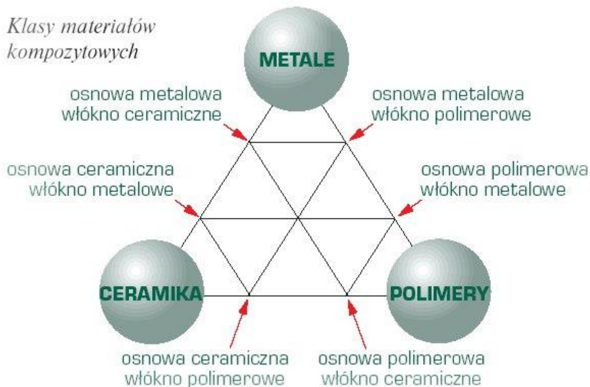
Rys. 1. Materiały kompozytowe. [8]
