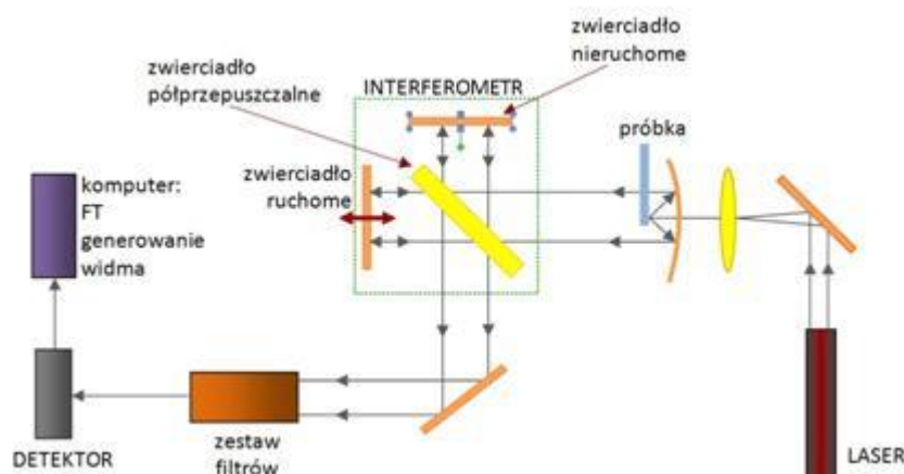
Rys. 4. Schemat spektrometru Ramana z transformacją Fouriera [1].
