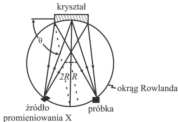
Rys. 3. Schemat monochromatyzacji metodą Rowlanda [1].
