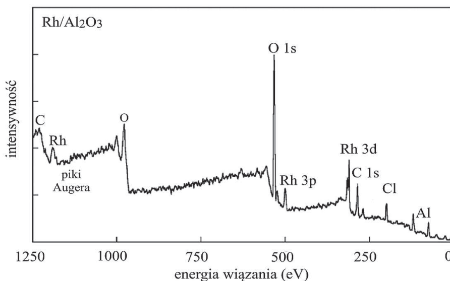
Rys. 6. Widmo XPS katalizatora Rh/Al 2 O 3 otrzymanego metodą impregnacji [1].
