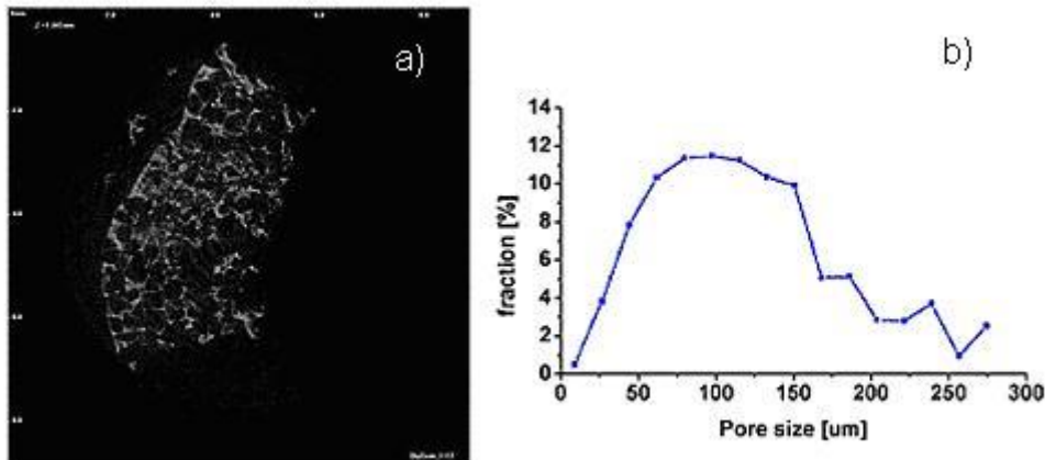
Rys. 6. Przekrój badanego rusztowania kostnego (a) oraz rozkład wielkości porów w tym rusztowaniu (b) (rozdzielczość 4.42 \mu\text{m} ).
