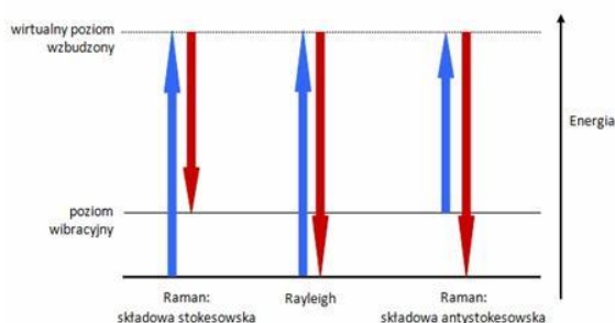
Rys. 1. Diagram energetyczny dla procesów rozproszenia Rayleigha i Ramana [1].
