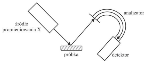
Rys. 2. Ogólny schemat aparatury do pomiarów metodą XPS [1].
