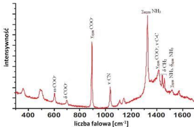
Rys. 2. Widmo Ramana glicyny (drgania: \nu -rozciągające, \delta -zginające, \gamma wahadłowe, \omega -wahlarzowe, sym -symetryczne, asym -asymetryczne) [1].
