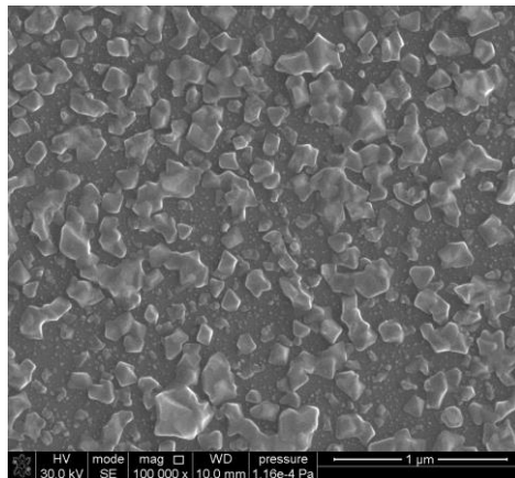
Rys. 3. Struktura ziaren miedzi o rozmiarach 200-500 nm wytwarzanych metodą CVD.
