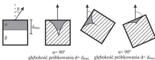
Rys. 7. Zmiana kąta zbierania elektronów ( \theta ) pozwala uzyskać widma pochodzące od pierwiastków znajdujących się na różnych głębokościach próbki [1].
