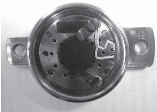
Rys. 5. Próbka katalizatora proszkowego, sprasowana w formę pastylki, zamontowana na nośniku reaktorowym [1].
