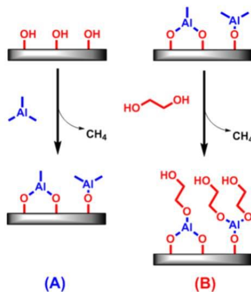
Rys. 7. Schemat wytwarzania organiczno-nieorganicznej monowarstwy hybrydowej metodą MLD.[13]
