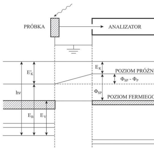
Rys. 1 Schemat poziomów energetycznych w próbce i spektrometrze [1].
