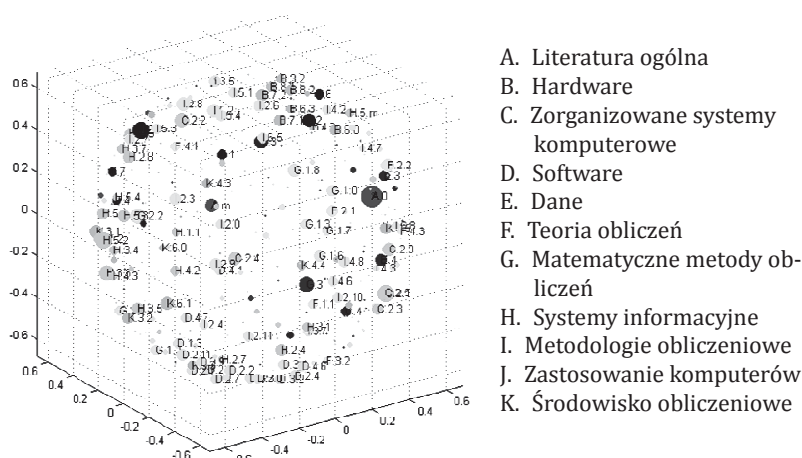
Rysunek 3. Klasy główne klasyfikacji CCS oraz ich graficzna reprezentacja na sferze (wg metody własnej)
