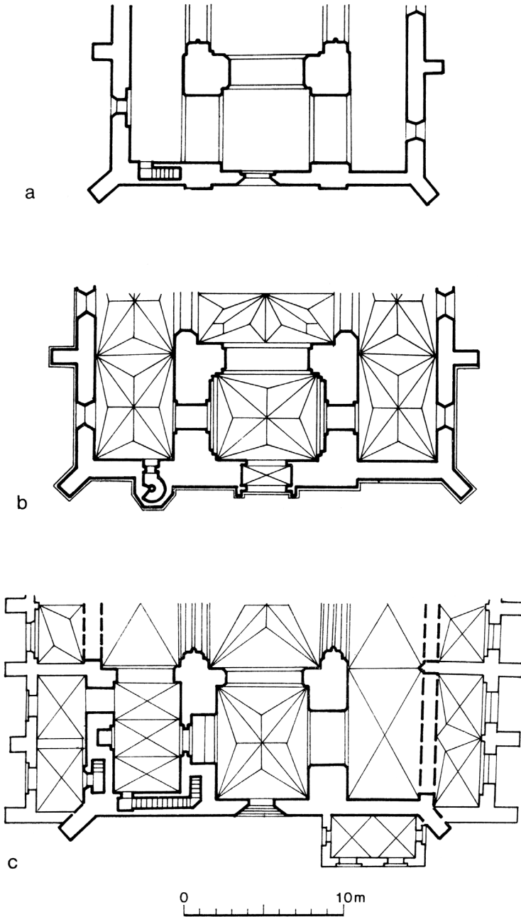
Il. 7. Rzuty masywów zachodnich jednowieżowych: a/ kościoła św. Mikołaja w Chelmży; b/ kościoła św. Mikołaja w Grudziądzu; c/ kościoła św. Jakuba w Toruniu, T. Mroczko, Architektura gotycka na ziemi chełmińskiej , Warszawa 1980, s. 189
